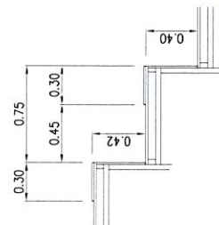
Particolare gradoni scala 1:25
